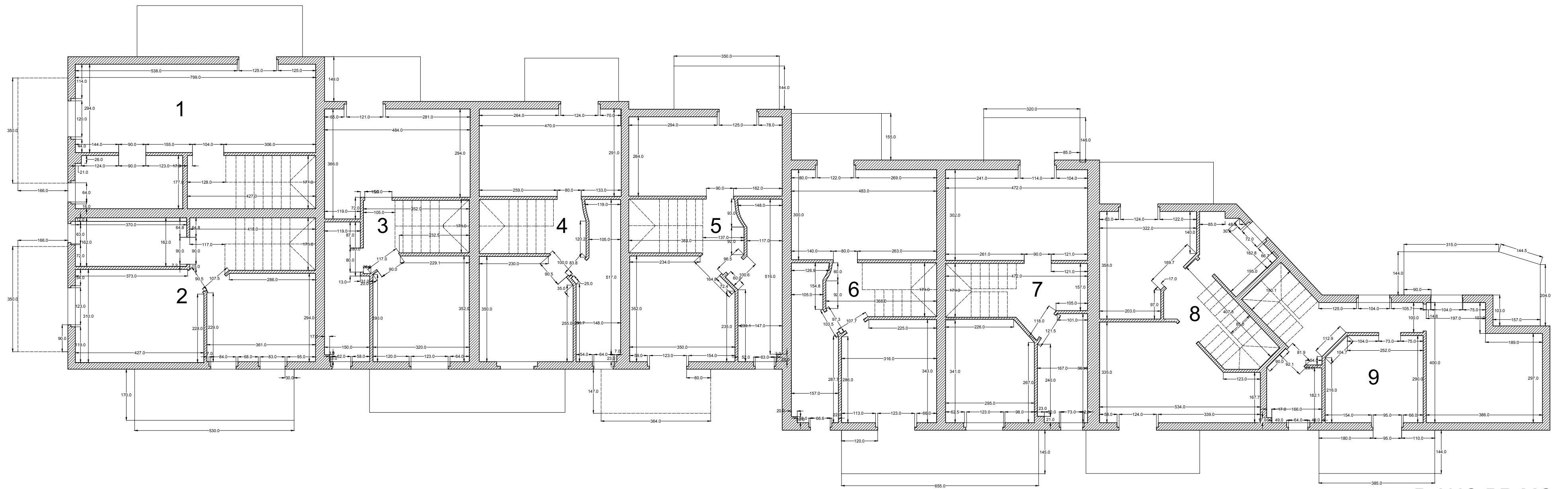
PIANO PRIMO
