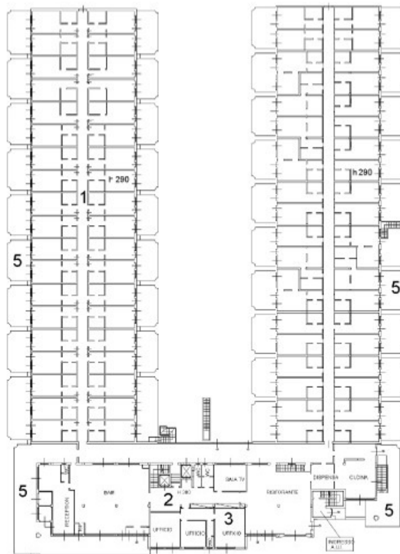
PIANTA PIANO TERRENO
