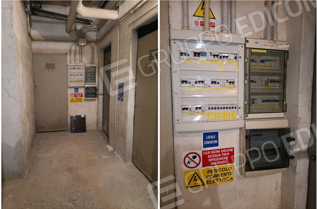
Quadri elettrici al piano seminterrato
