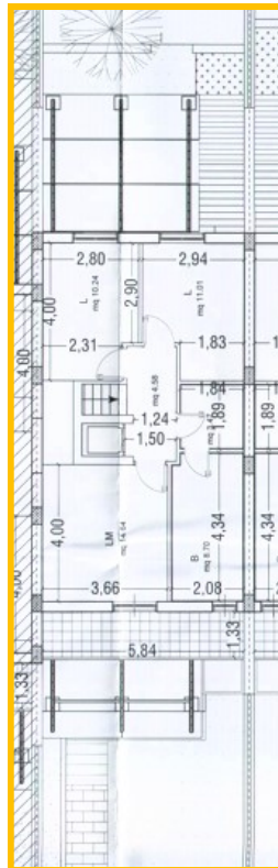
Pianta di progetto P.1°
