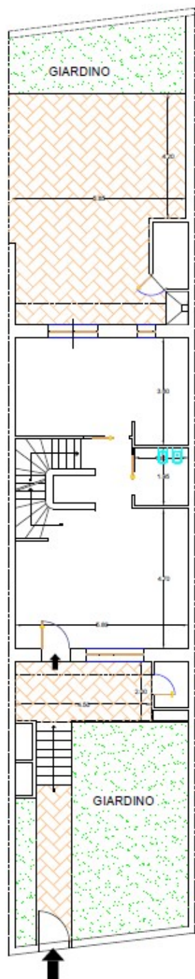
PIANTA PIANO TERRA Fg. 50 pat. 2891 sub 3
