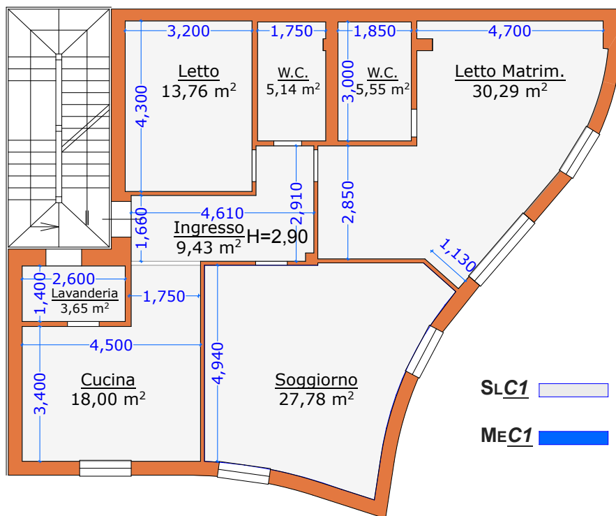
PIANTA QUOTATA APPARTAMENTO C1
