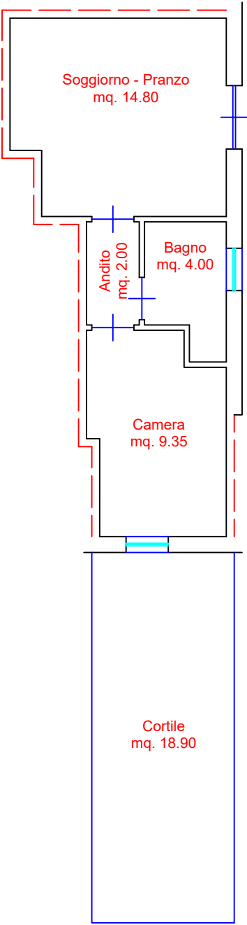
PIANO TERRA PLANIMETRIA STATO DI FATTO SCALA 1:100
