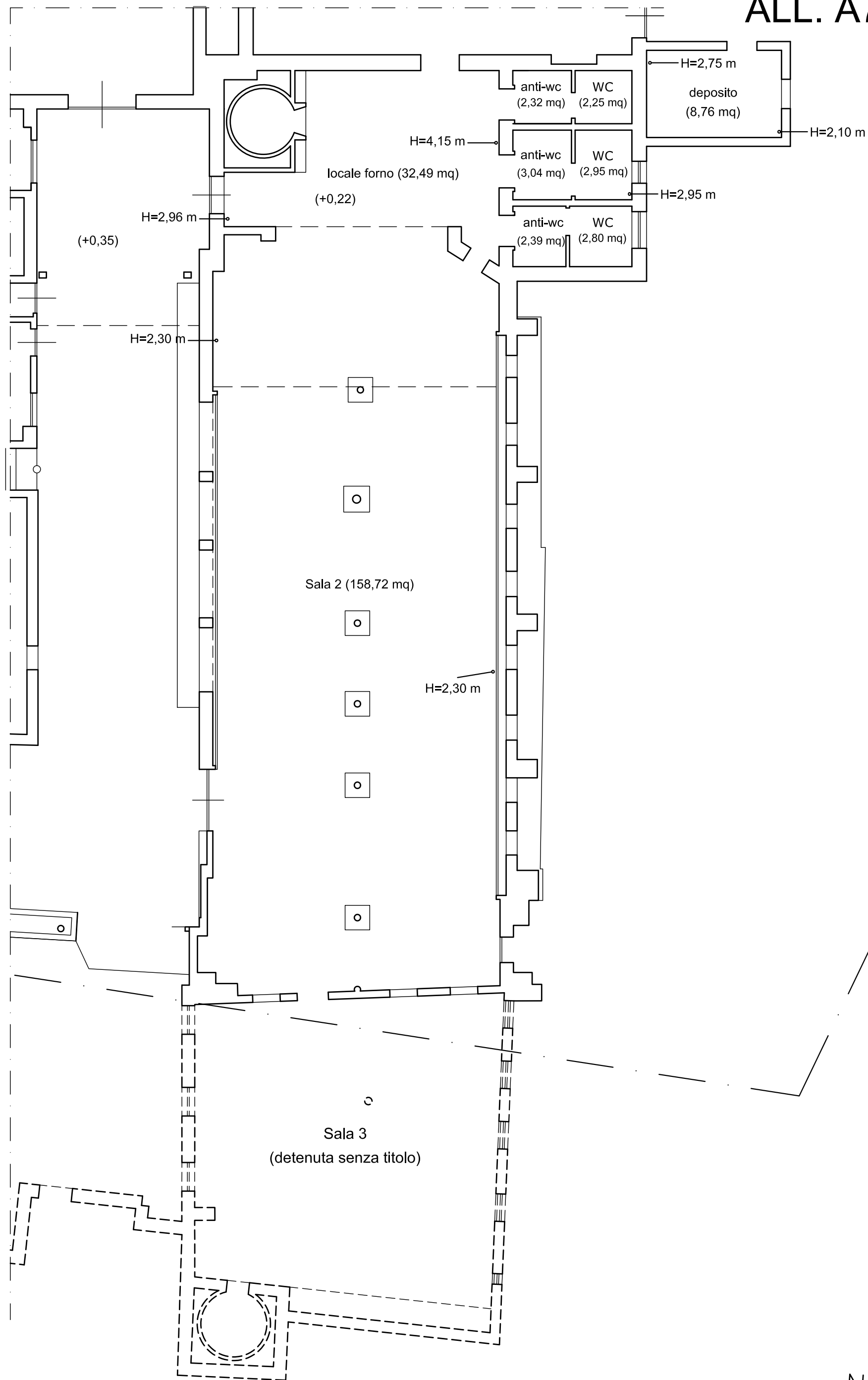
Planimetria edificio 3 (Locali realizzati in assenza di titolo edilizio)
