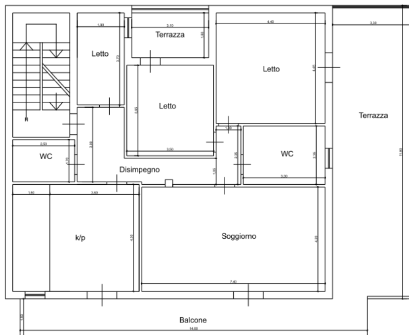
Fig.8: rilievo planimetrico dei locali
