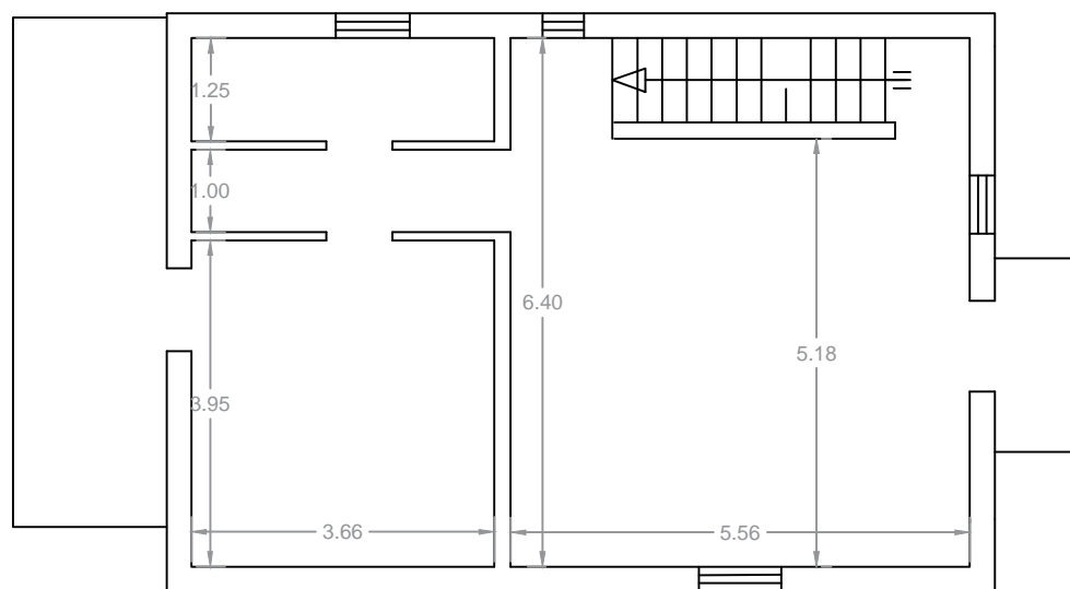
Pianta piano Primo H= 3.00 m
