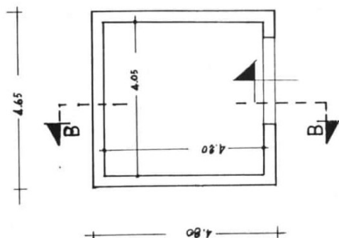
PIANTA MAGAZZINO
