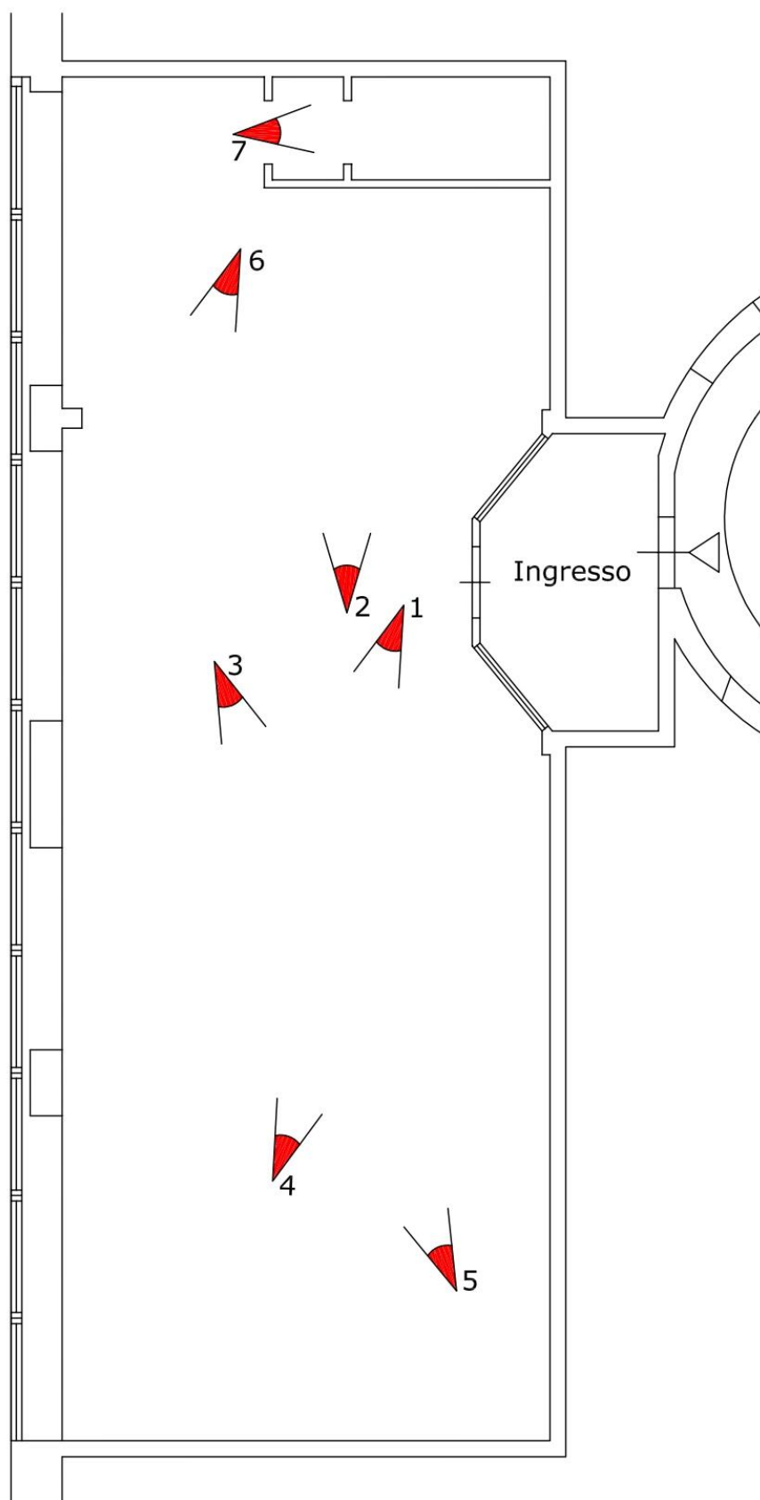
PLANIMETRIA CONI OTTICI
