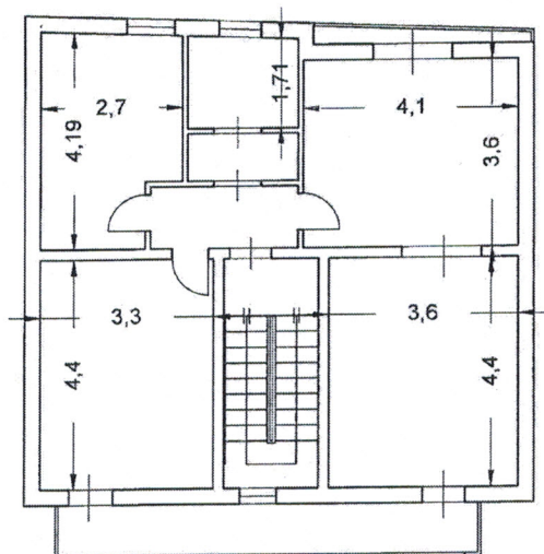
Planimetria stato di fatto scala 1:100
