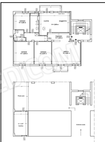
Rilievo
