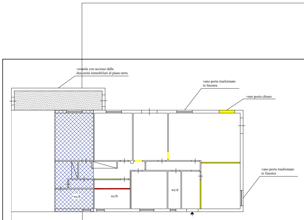
Schema grafico con difformità tra lo stato di fatto e la planimetria catastale
