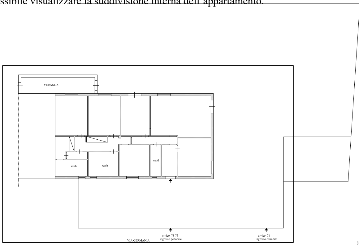
Schema grafico di rilievo
