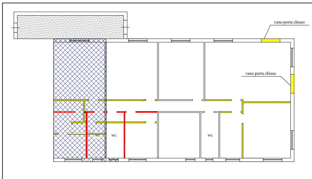
Schema grafico che evidenzia le difformità planimetriche tra lo stato di fatto e la planimetria di progetto
