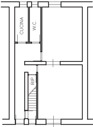
PIANO TERRA H. mt. 2.85
