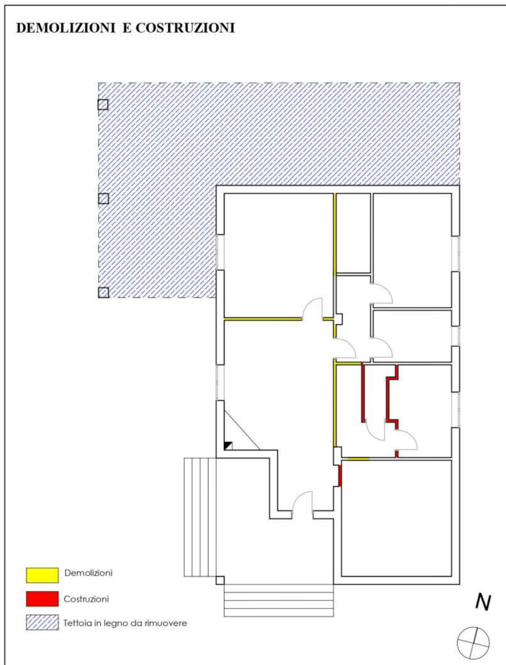
Rilievo attuale dei luoghi con indicazione grafica delle difformità ( demolizioni e ricostruzioni) (All. 5.1)
