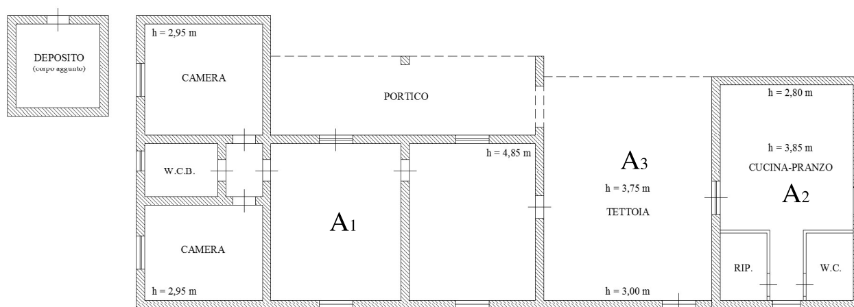
CORPO A - Abitazione (Part.III 184/7 - P.T.) - Scala 1:100
