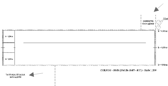
Rilievo stato attuale dei luoghi (sub. 5)
