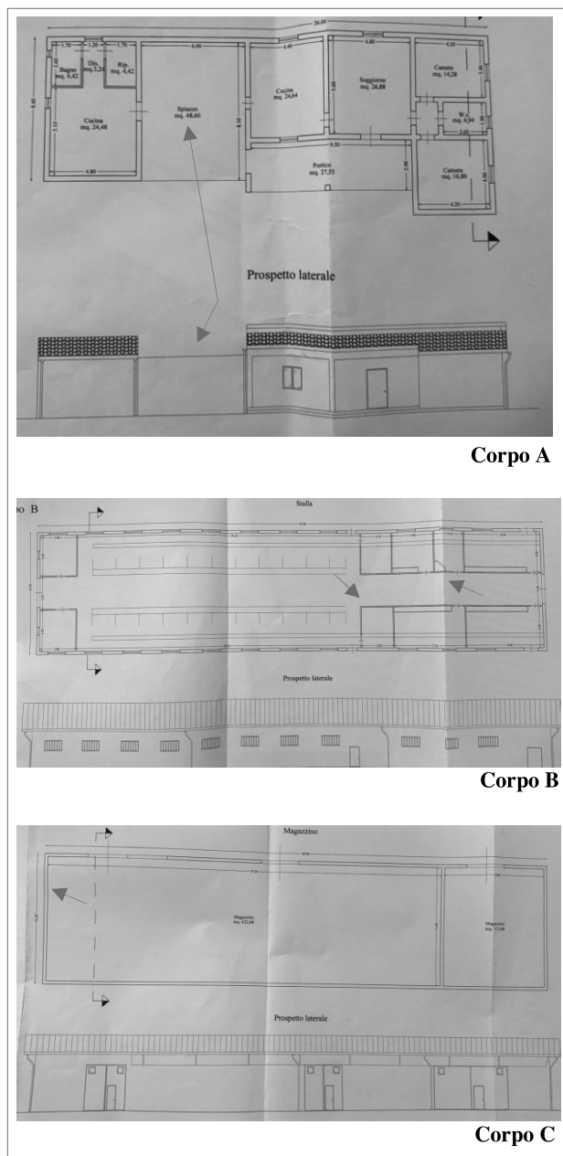
Stralci progettuali reperiti c/o U.T.C. raffiguranti lo stato attuale
