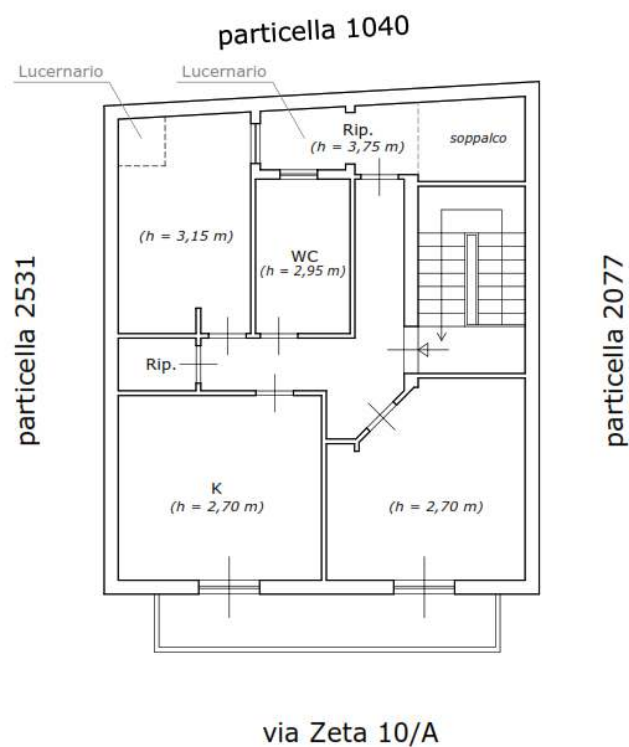
Rilievo planimetrico dell'immobile
