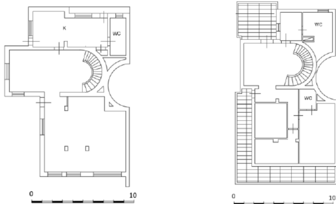
Planimetria di rilievo attuale piano terra e piano primo (All. 6)
