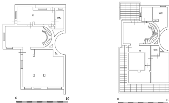
Rilievo dello stato dei luoghi piano terra e piano primo (All. 6)
