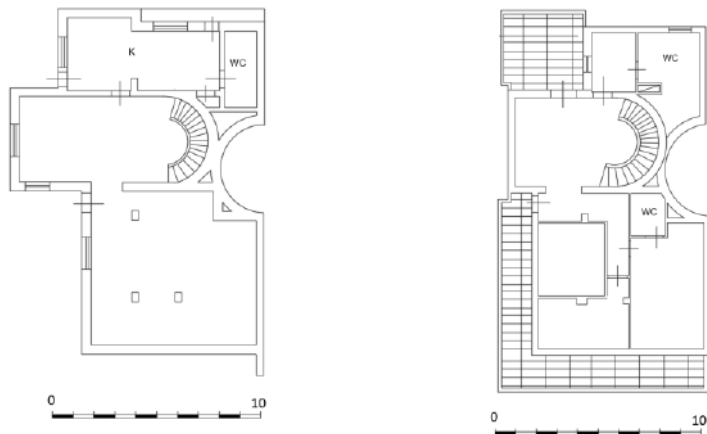
Ricostruzione planimetria catastale piano terra e piano primo (All. 9)
