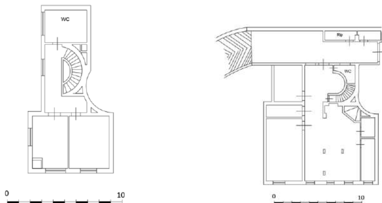
Planimetria dello stato futuro piano secondo ed S1 (All. 9)
