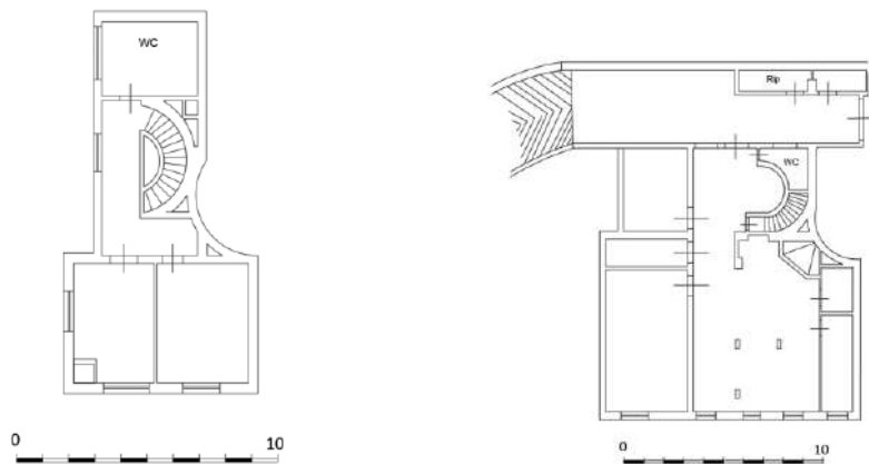
Ricostruzione planimetria catastale piano secondo ed S1 (All. 9)
