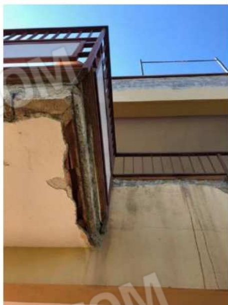
ammaloramenti sotto balconi, pilastri e
