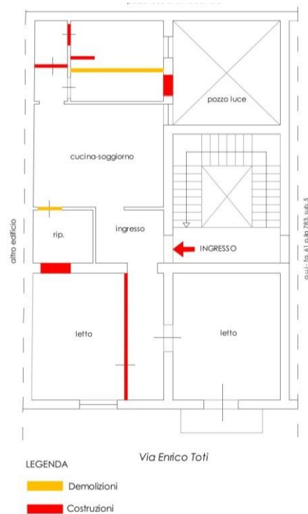
Planimetria di rilievo attuale con indicazione delle difformità rispetto al grafico di progetto allegato alla licenza edilizia n. 881 del 1958.
