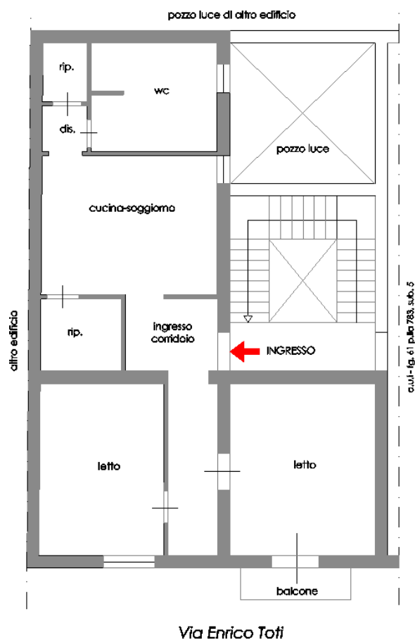
Planimetria di rilievo dello stato di fatto reale dei luoghi (All. B1)
