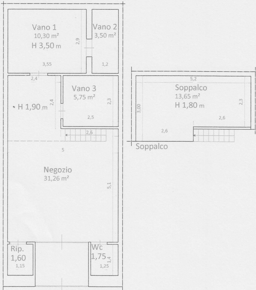
Via Abramo Lincoln 31 PIANTA NEGOZIO
