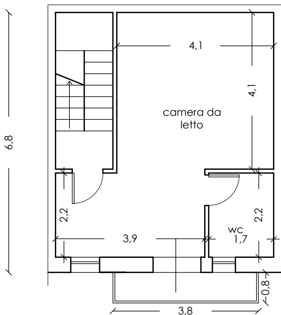
Piano Primo stato di fatto
