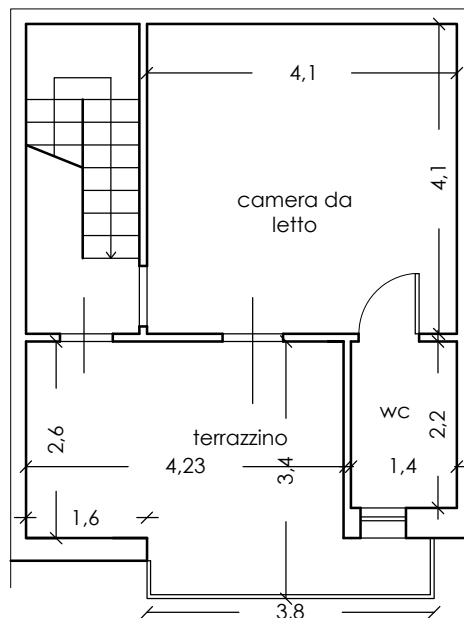
Piano Secondo stato di fatto
