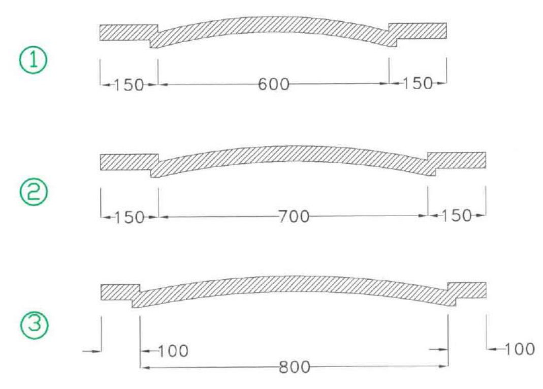
SEZIONI STRADALI TIPO
