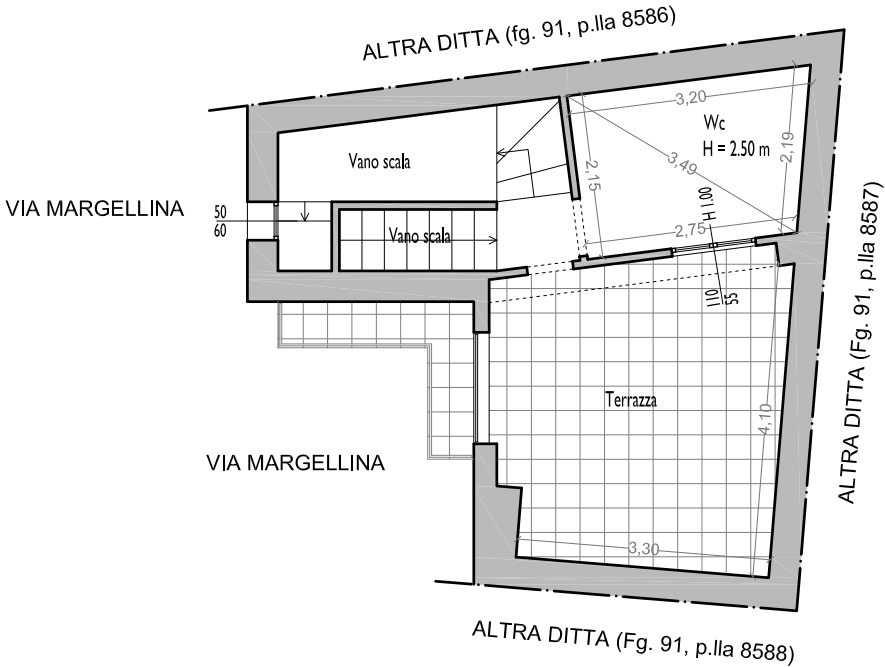
rilievo STATO DI FATTO piano terrazza scala 1:100
