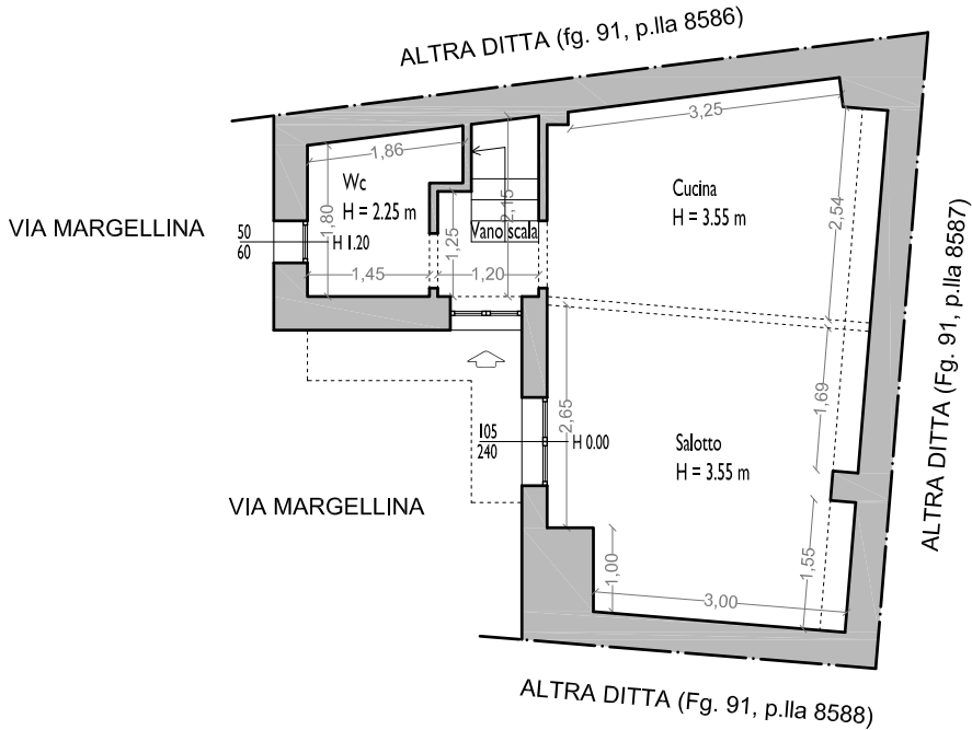
rilievo STATO DI FATTO piano terra scala 1:100
