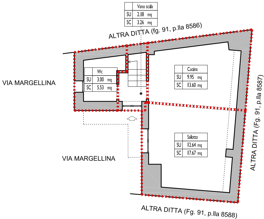
calcolo SUPERFICIE COMMERCIALE piano terra scala 1:100
