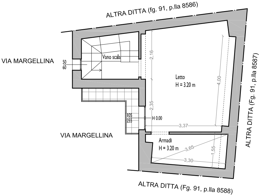
rilievo STATO DI FATTO piano primo scala 1:100
