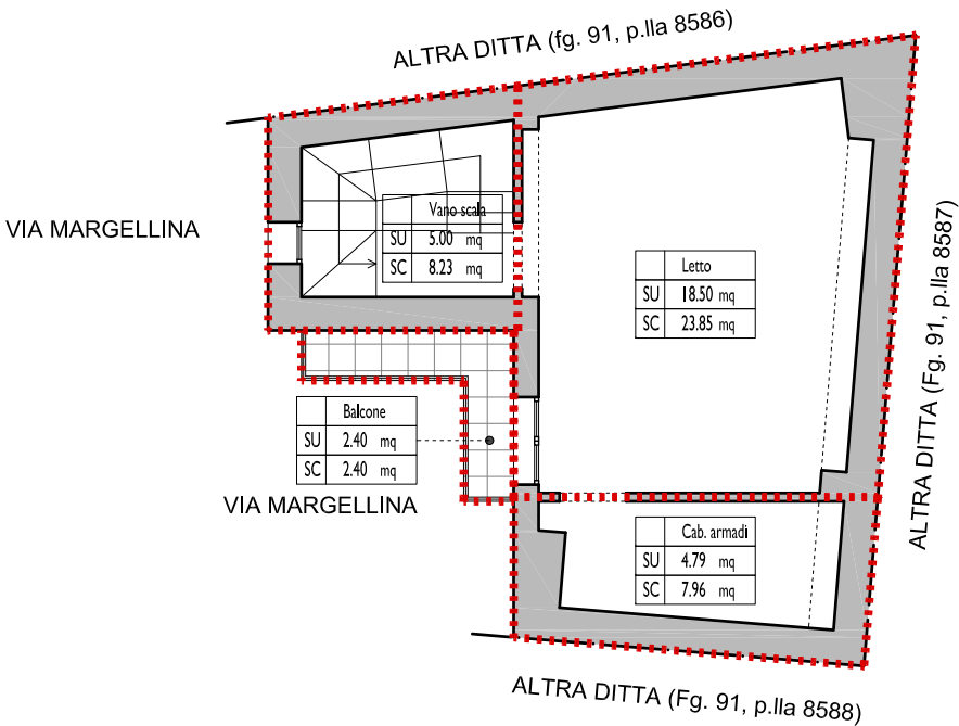
calcolo SUPERFICIE COMMERCIALE piano primo scala 1:100
