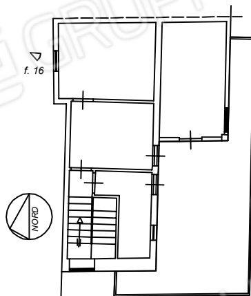
pianta piano terzo e copertura
