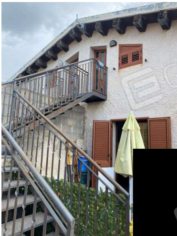
Foto 5: Vista prospetto esposto a Ovest, si fa notare che la finestra al piano sottotetto è difforme rispetto al prospetto approvato con C.E. in Sanatoria n° 161/2000, e non è regolarizzabile, pertanto è da murare. Anche la scala in ferro di accesso al piano sottotetto non risulta negli elaborati di progetto e se ne prevede la rimozione.
