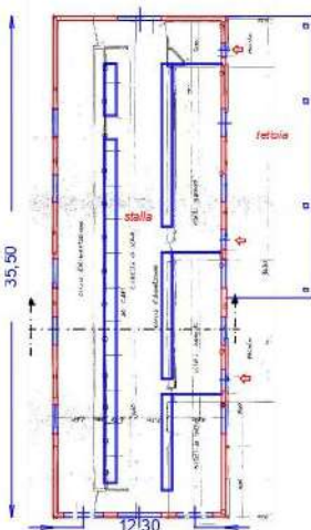
sovrapposizione tra stato di fatto e planimetria allegata alla C.E. del 1985
