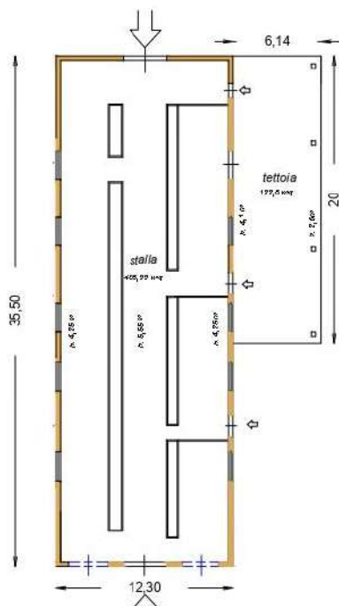
PLANIMETRIA RILEVATA
