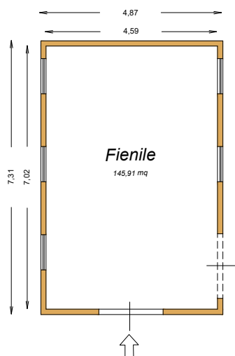
PLANIMETRIA RILEVATA
