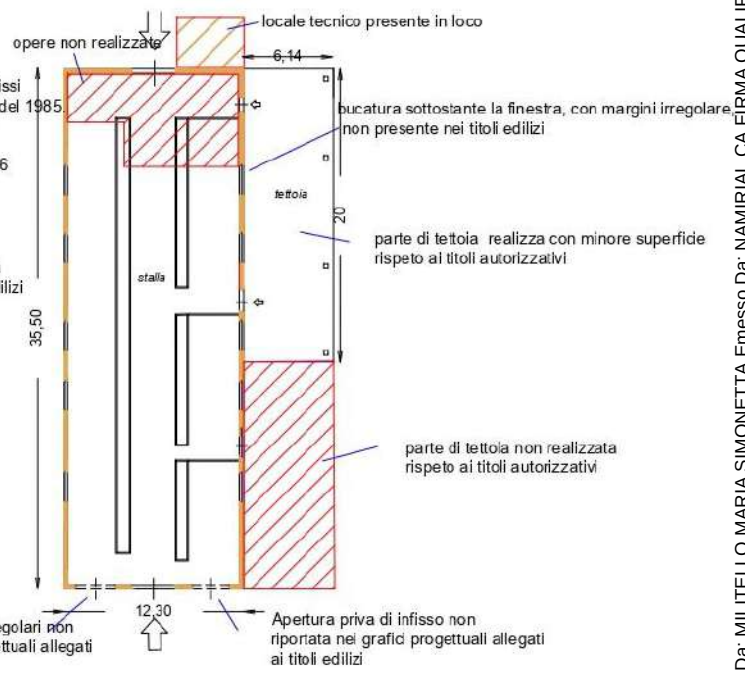
PLANIMETRIA RILEVATA -indicazioni delle difformità
