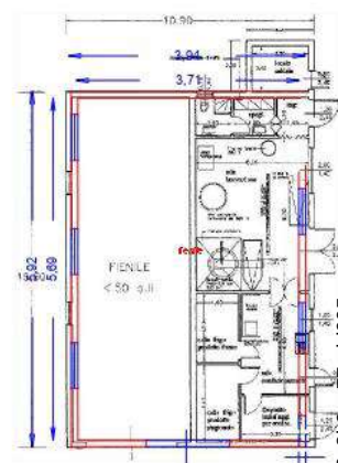
sovrapposizione tra stato di fatto e stato di progetto allegato al PDC del 2016
