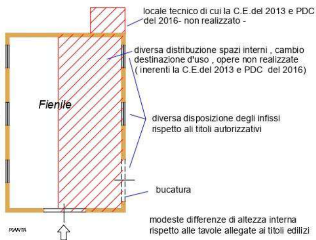
PLANIMETRIA RILEVATA -indicazioni delle difformità
