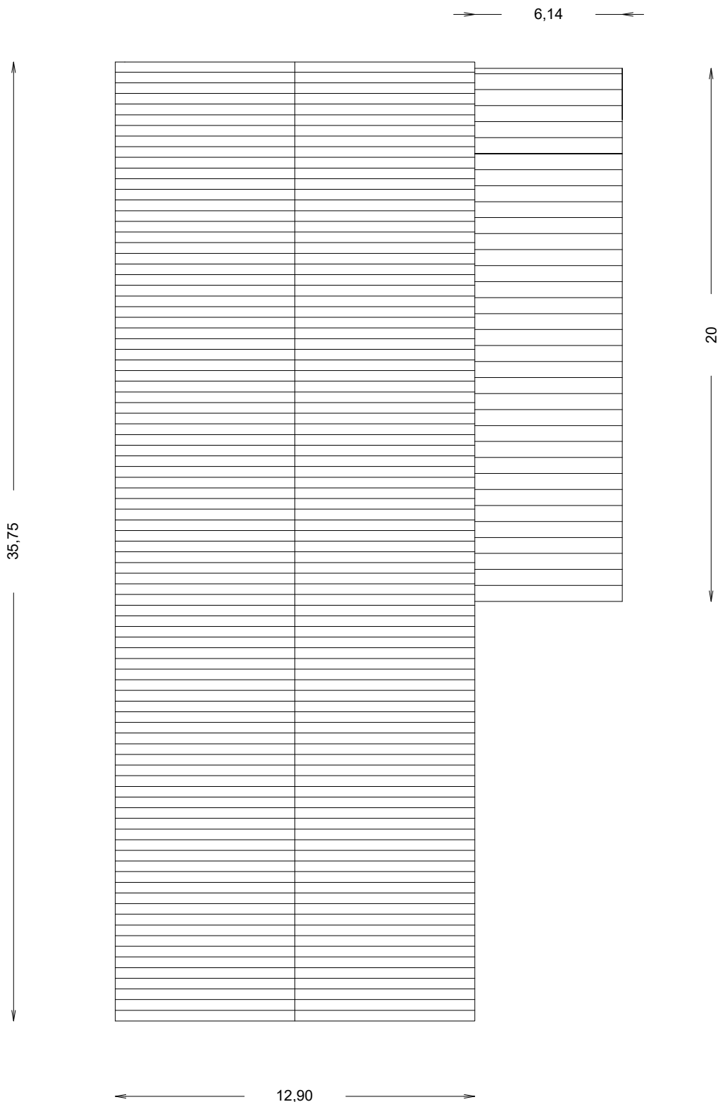
PIANTA DELLA COPERTURA
