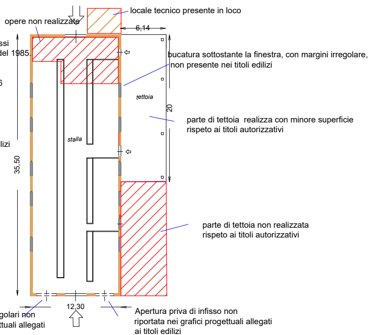
PLANIMETRIA RILEVATA -indicazioni delle difformità
