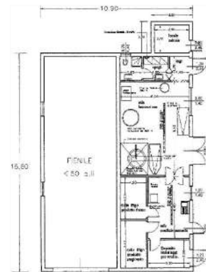
variante di progetto allegato al PDC 2016
