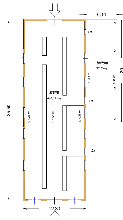
PLANIMETRIA RILEVATA
