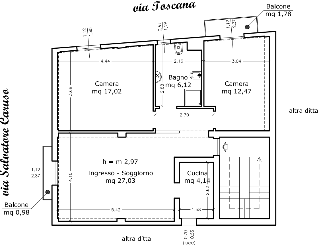
Piano terzo
