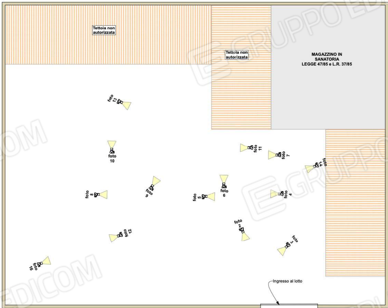
Planimetria lotto con coni ottici - scala 1:200
