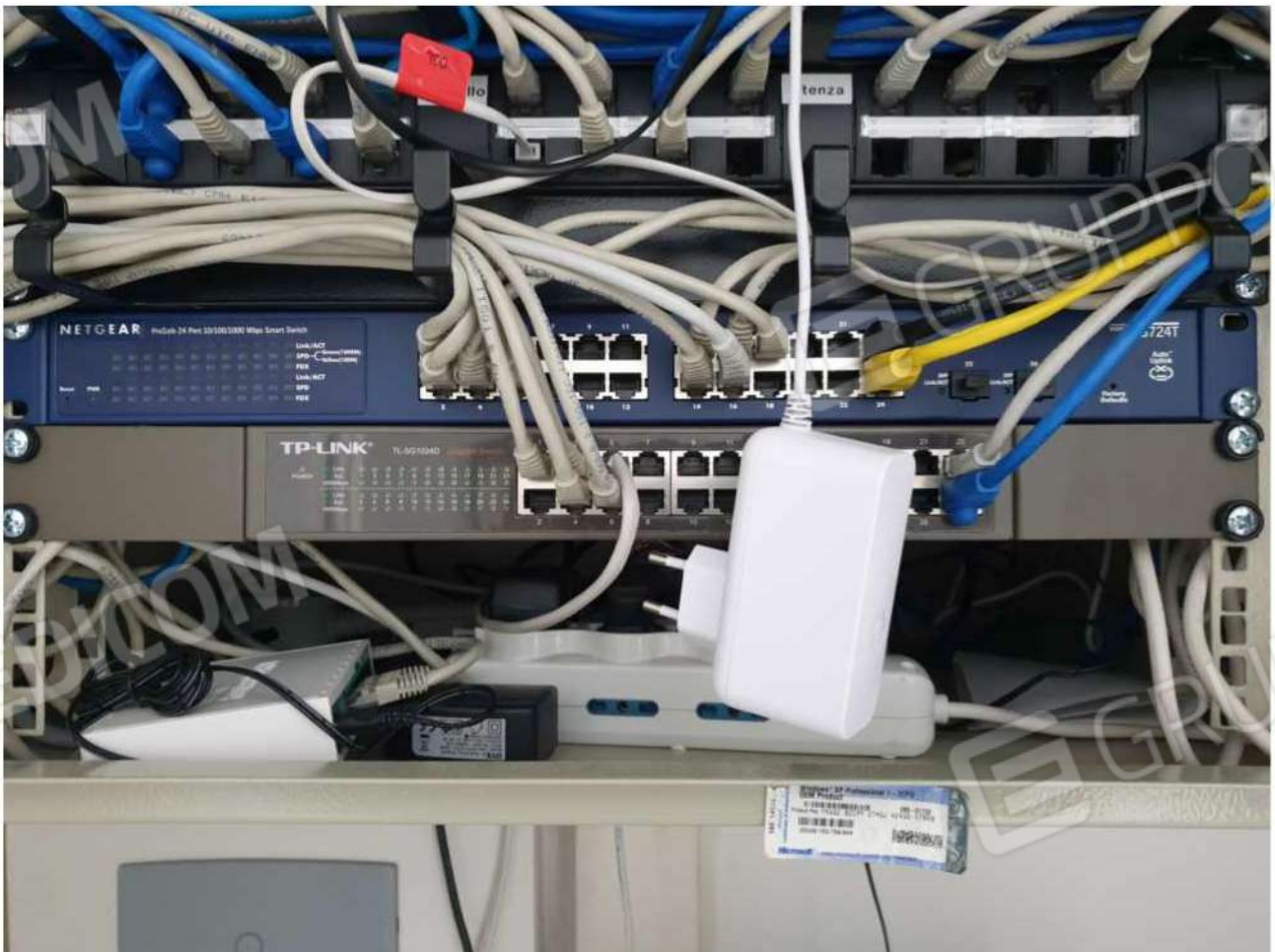
Foto 23 e 24. Ufficio 1, rastrelliera informatica (rack) composto da Fireworlds marca Netgear ProSafe 24 porte (Model GS724T), Switch marca TP-LINK modello TL-SG1024D, pannello telefonico e n° prese universali
