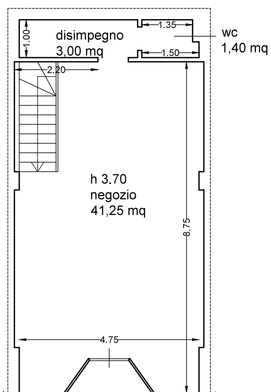
Planimetria piano terra 1:100 stato rilevato
