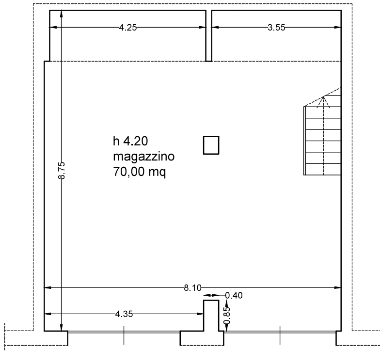
Planimetria piano S1 1:100 stato rilevato
