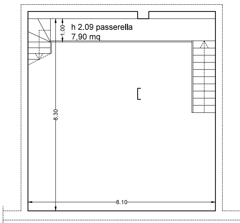
Planimetria passerella 1:100 stato rilevato
