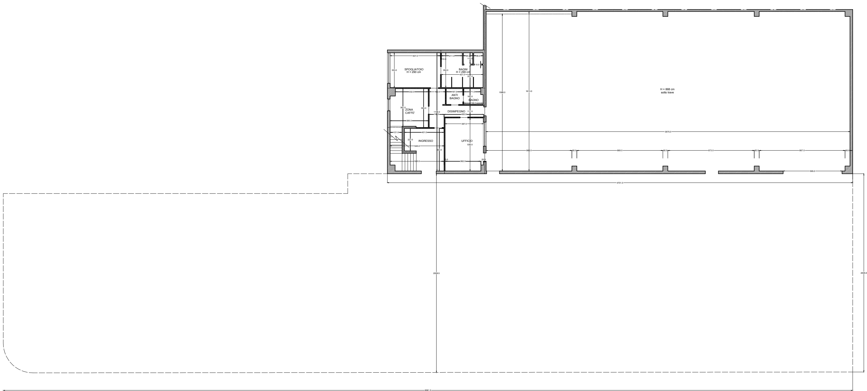
PIANTA PIANO TERRA CON ESTERNO
