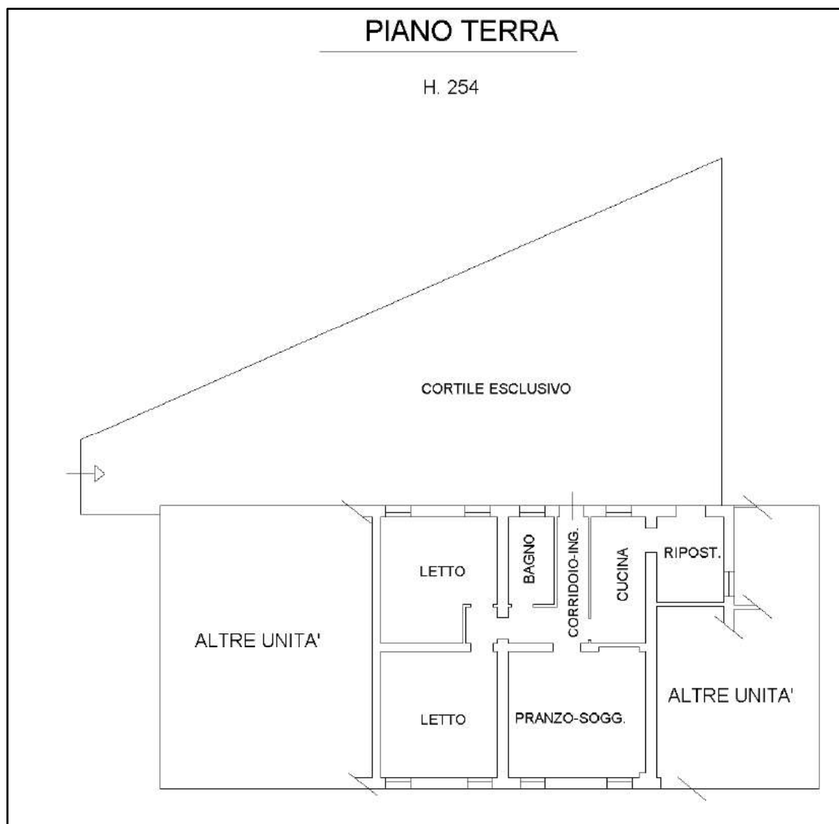
Figura 5 – Planimetria subalterno 10 (soppresso)
