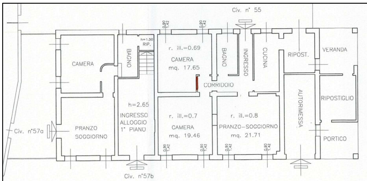
Figura 18 - Estratto dalla DIA n. 195/99 – Stato di progetto
