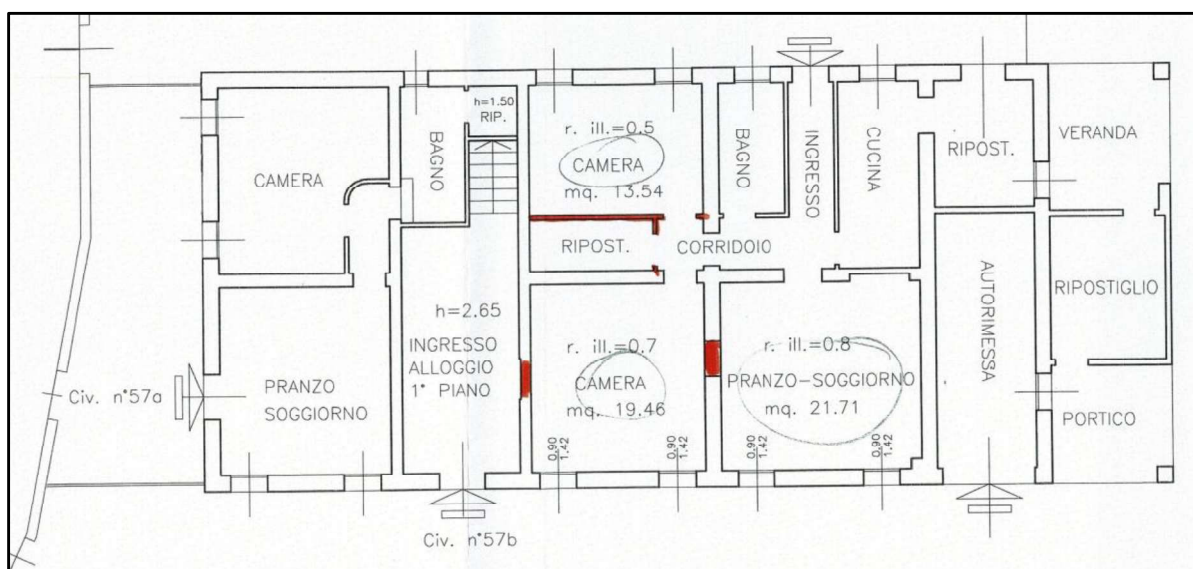
Figura 17 – Estratto dalla DIA n. 195/99 – Stato di progetto (in rosso pareti da costruire)
