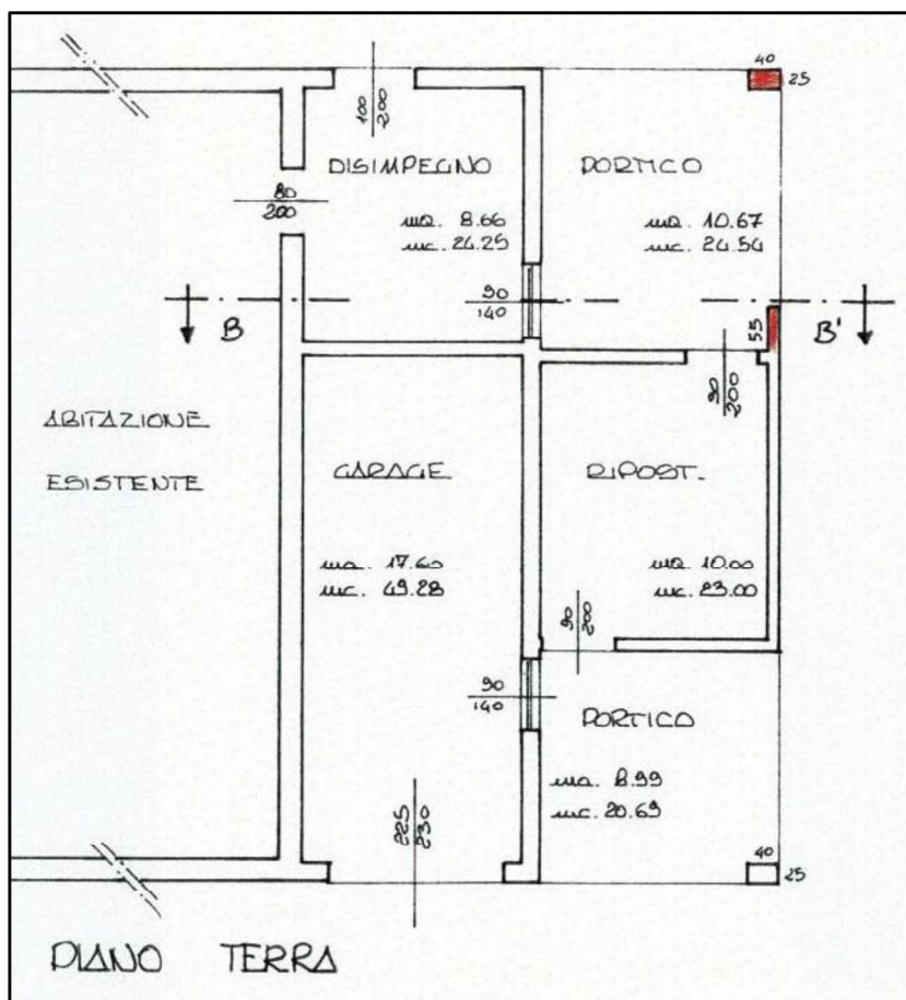
Figura 20 – Estratto dalla C.E. n. 28/93
