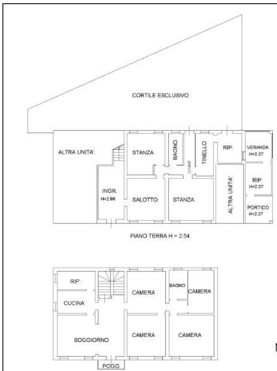
Figura 3 – Estratto della planimetria catastale del subalterno 13
