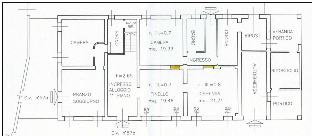
Figura 16 – Estratto dalla DIA n. 195/66 – Stato di fatto (in giallo pareti da demolire)
