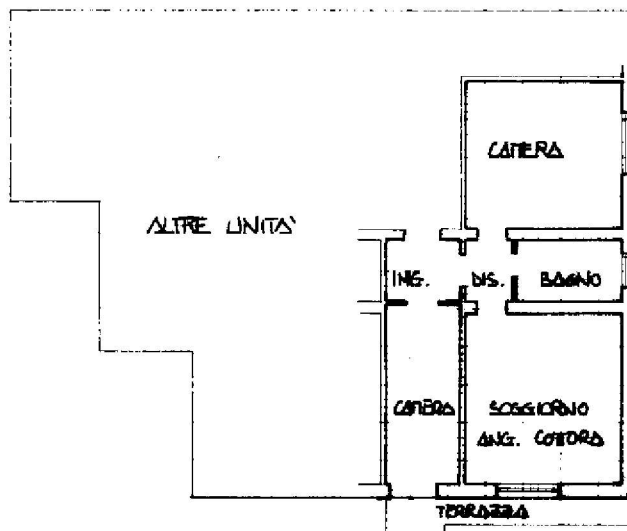
PIANTA PIANO PRIMO H=2.90
