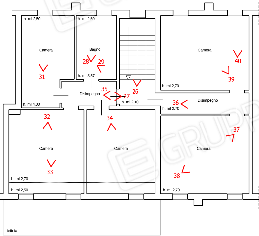
Piano Primo
