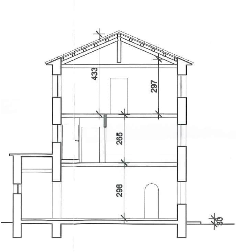
SEZIONE A-A
