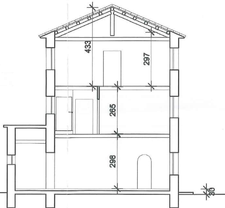
SEZIONE A-A
