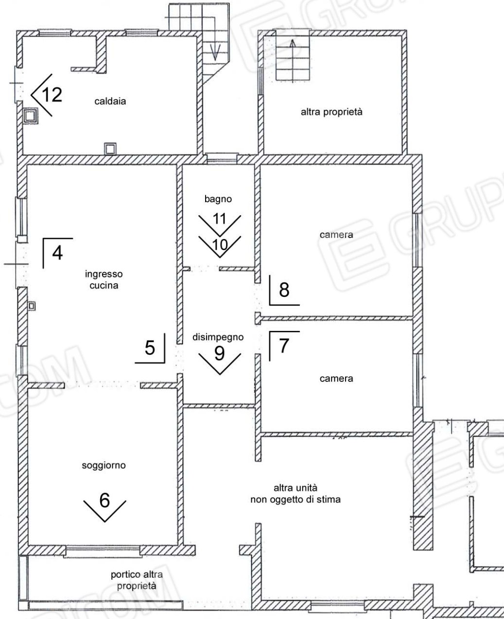
PLANIMETRIA IN SCALA 1:200
