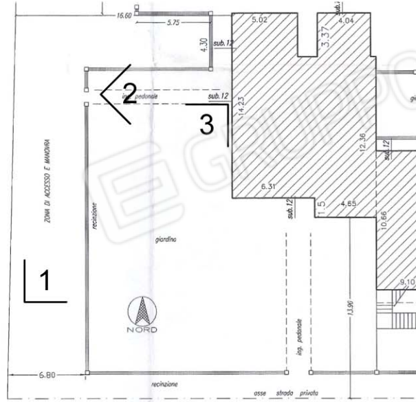
PLANIMETRIA IN SCALA 1:200
