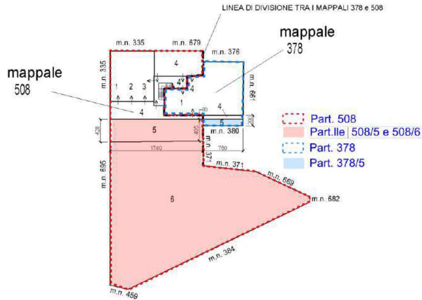
ESTRATTO ELABORATO PLANIMETRICO 2007
