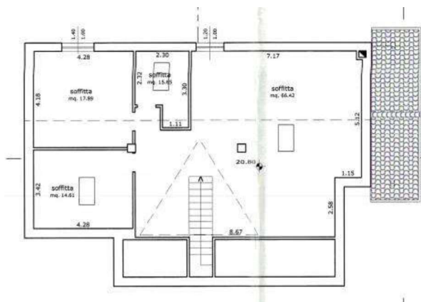
ESTRATTO PDC 97E DEL 18.06.2007 - PIANO SOTTOTETTO
