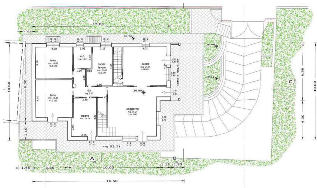
ESTRATTO PDC 97E DEL 18.06.2007 - PIANO TERRA
