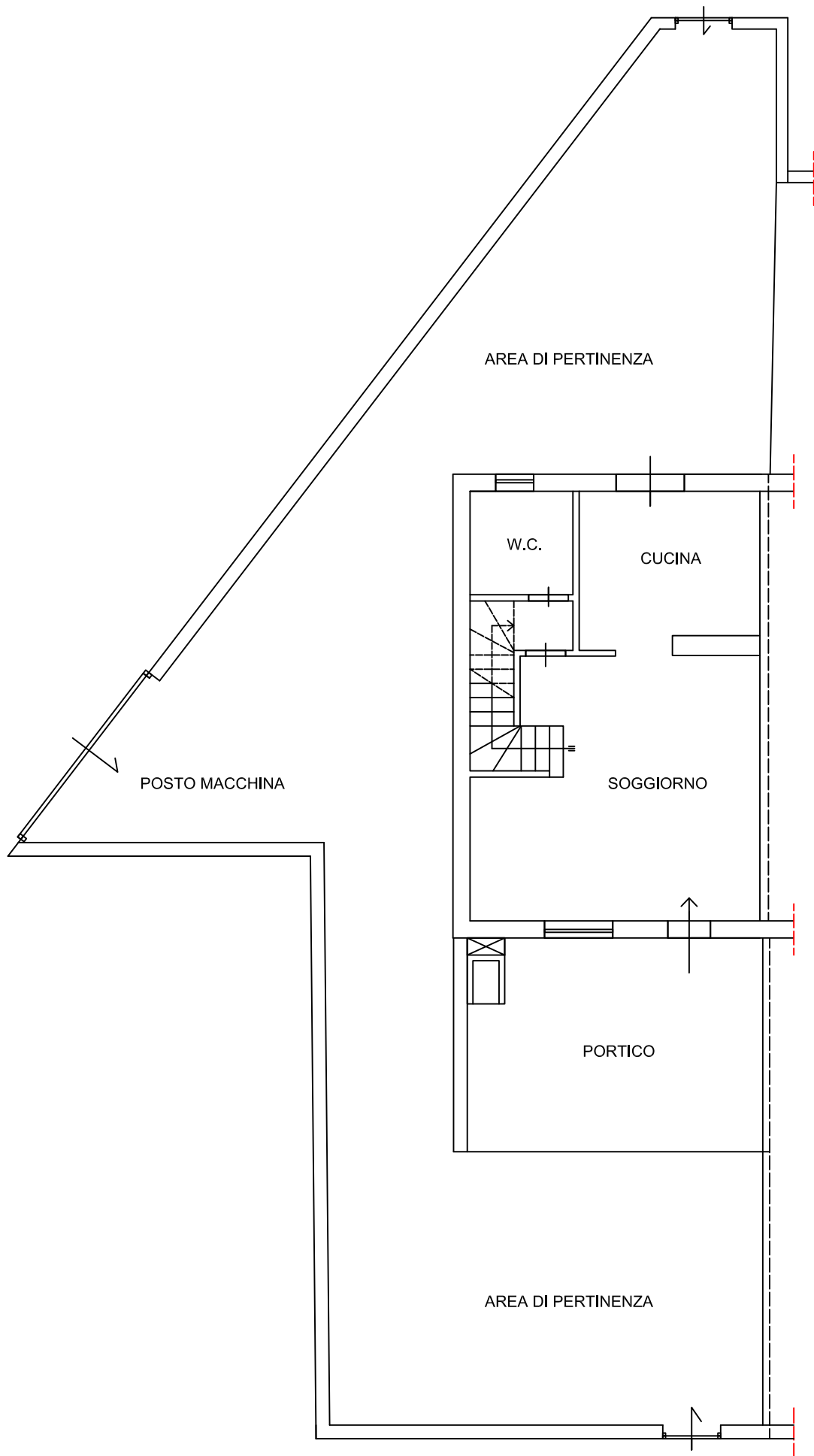
PIANTA PIANO TERRA DA RILIEVO EFFETTUATO
