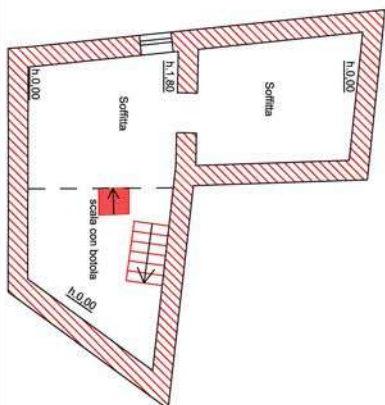
PLANIMETRIA RILEVATA PIANO TERZO (SOFFITTA)
