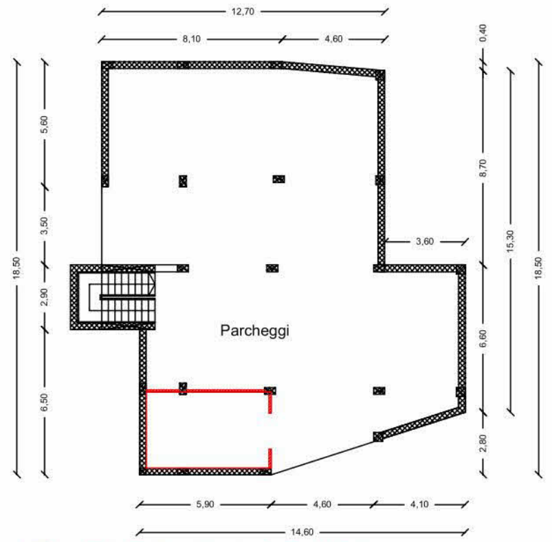
PIANTA PIANO INTERRATO STATO DI FATTO
