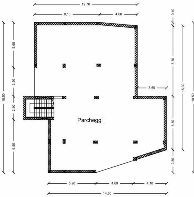
PIANTA PIANO INTERRATO STATO DI PROGETTO
