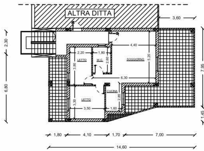
PIANTA PIANO SECONDO STATO DI PROGETTO
