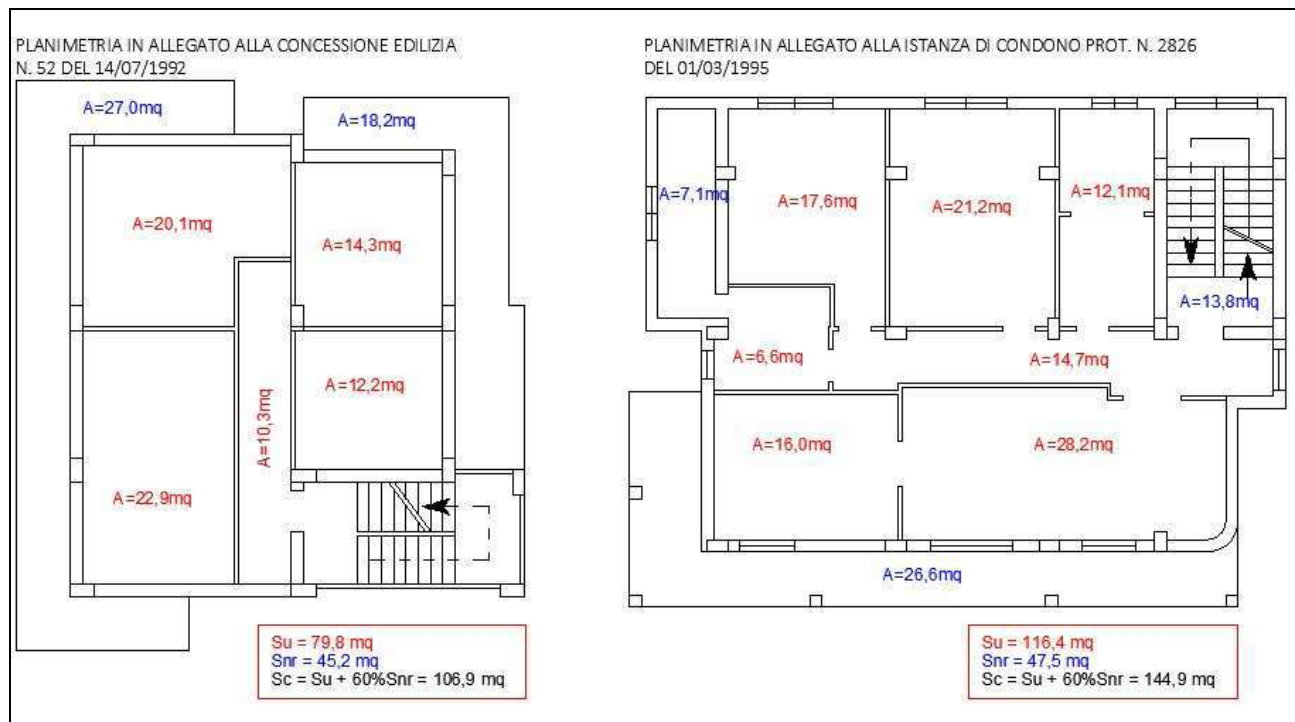
Fig. 13: Planimetrie dell'immobile allegate rispettivamente alla concessione edilizia n. 52 del 14.07.1992 e ed alla istanza di condono prot. n. 2826 del 01/03/1995, con indicazione delle superfici.
