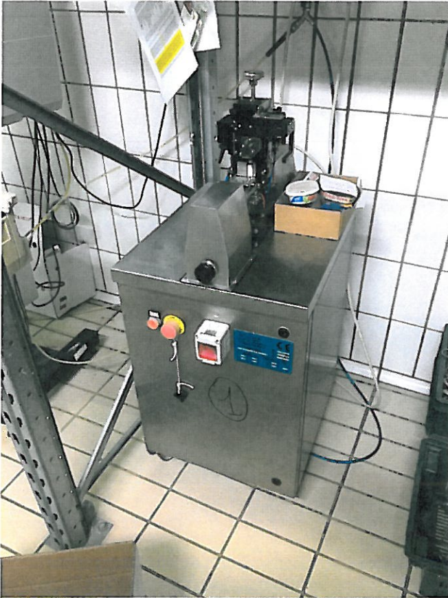
MACCHINA PER SIGILLI
