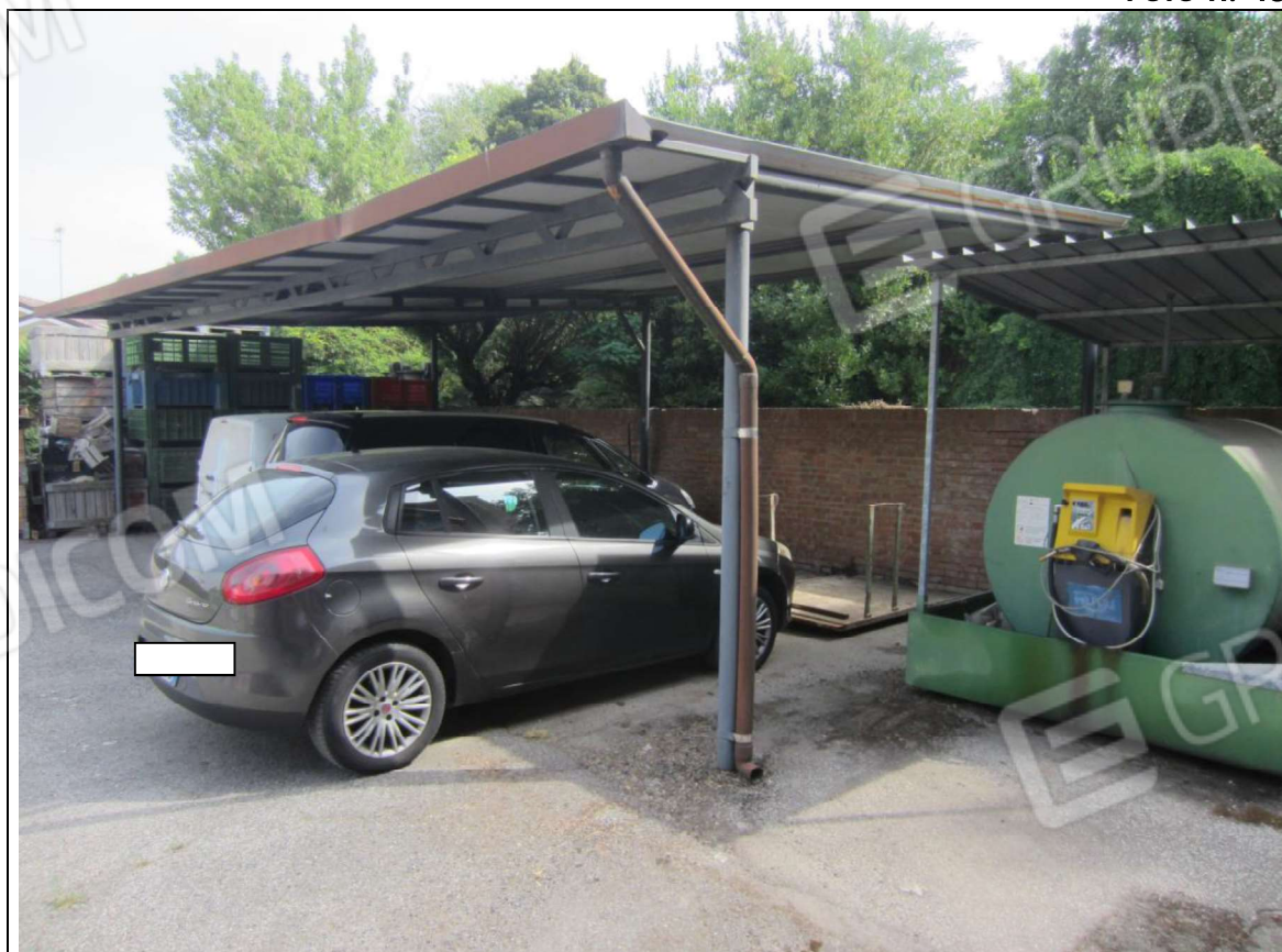
TETTOIA METALLICA MAPP. 239 SUB 9
