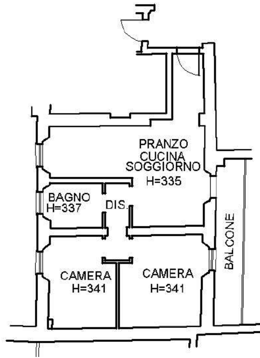
estratto dalla planimetria catastale attuale dell'appartamento
