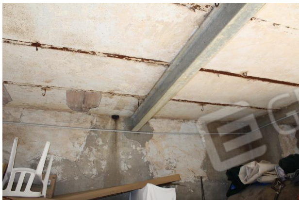
PARTICOLARE RINFORZI IN ACCIAIO AL SOLAIO PIANO PRIMO
