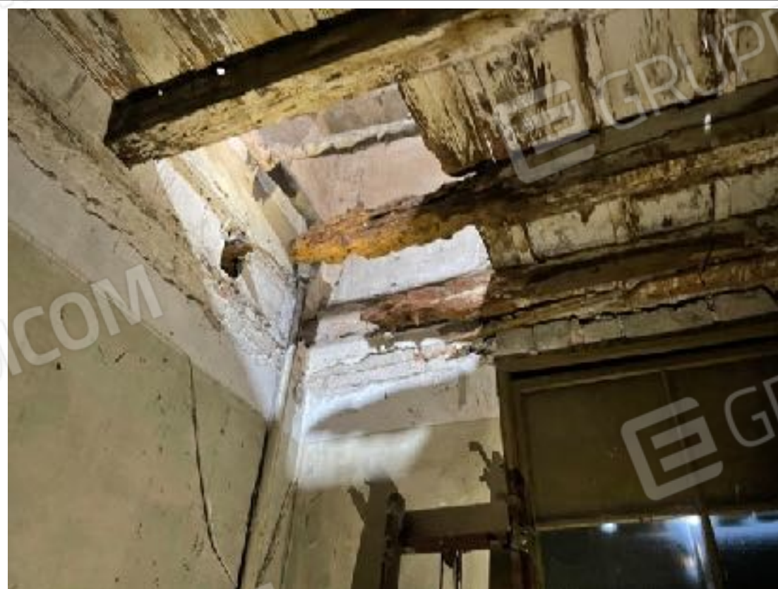
Particolare solai ammalati piano secondo
