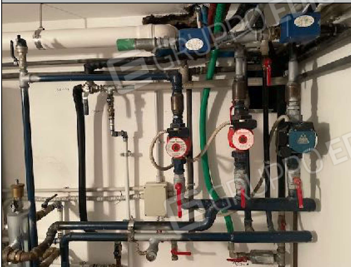
Centrale termica: particolare tubature caldaia
